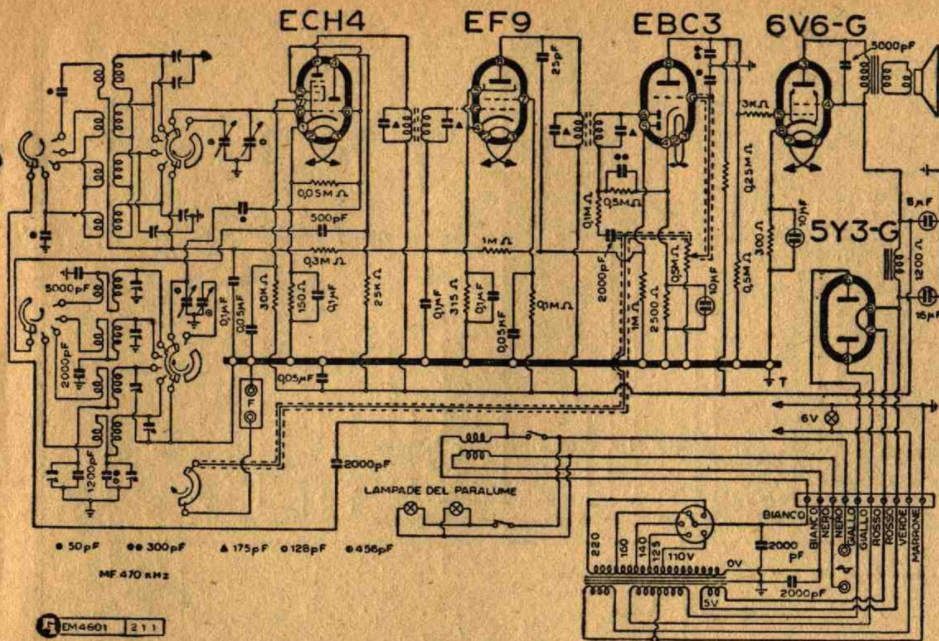
Lo schema del mod. 546 B realizzato nella radiolampada.
